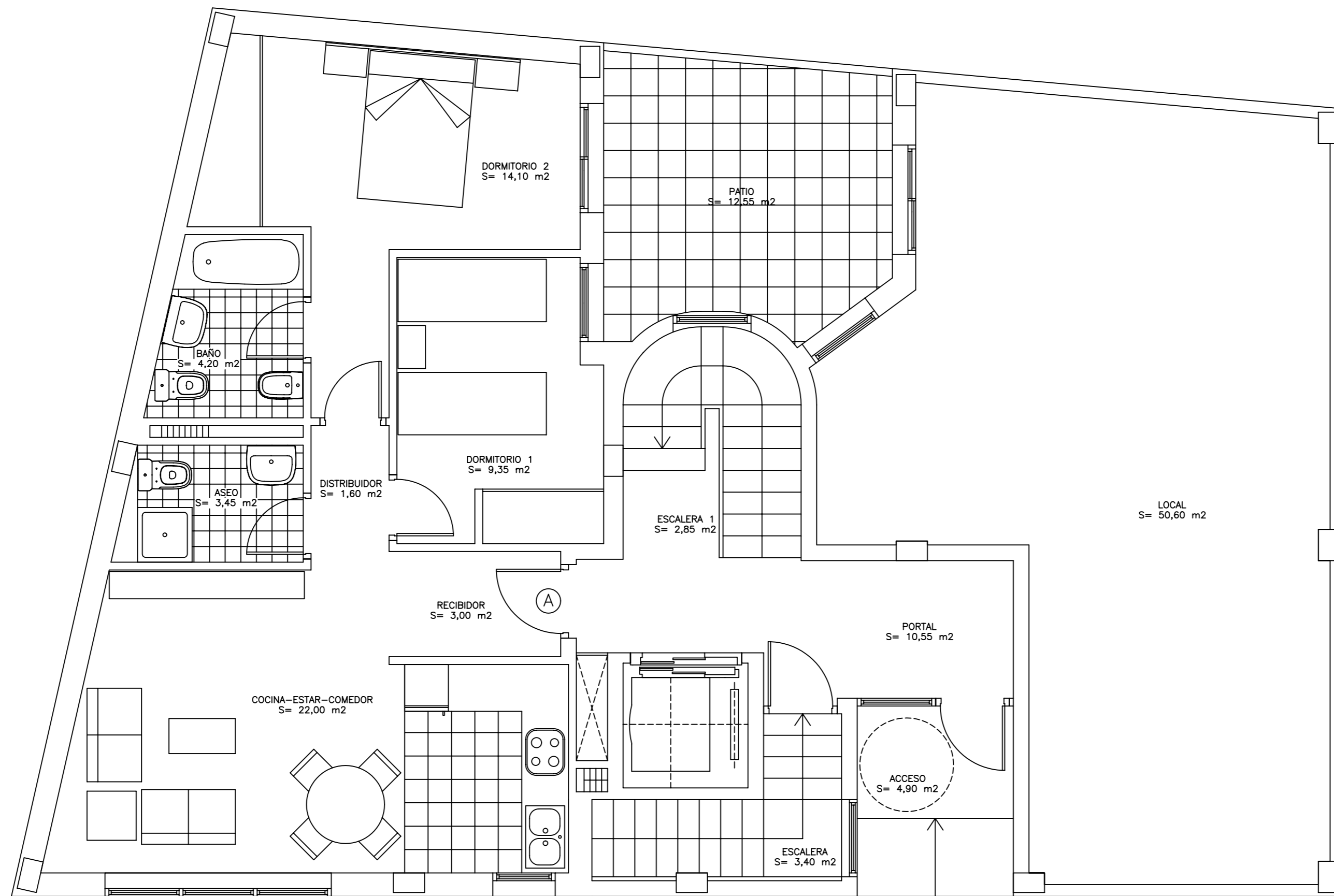
PLANTA BAJA. COTA ±0,00. DISTRIBUCIÓN Y SUPERFICIES.
